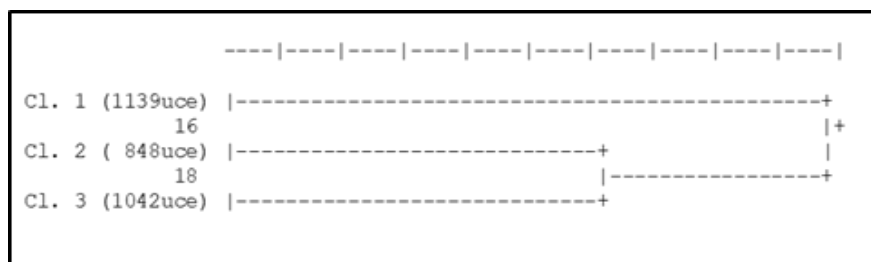
Figure 1_ Dendrogramme livré par le logiciel Alceste
